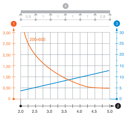
Belastingssdiagramm Kabelleiter Typ L 110 VS
