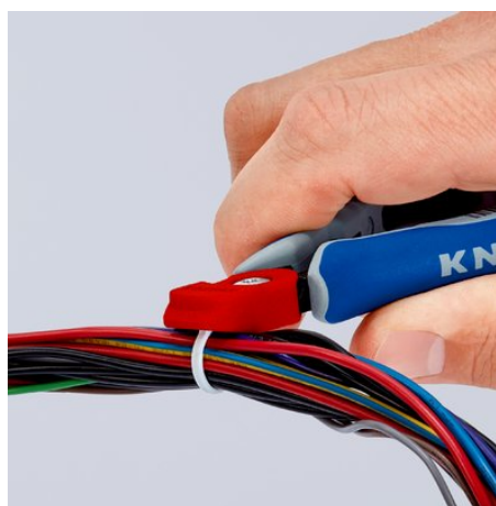
Usuń główkę opaski zaciskowej za pomocą szczypiec tnących bocznych dla elektroników...
