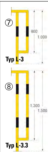
Gütestahlbügel in halbrunder Form zum Schutz gegen Anfahrsschäden, Rohrdurchmesser 48 mm
