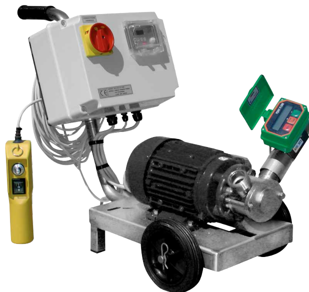
NIROSTAR 2000-C mit Frequenzumrichter und Fernbedienung
