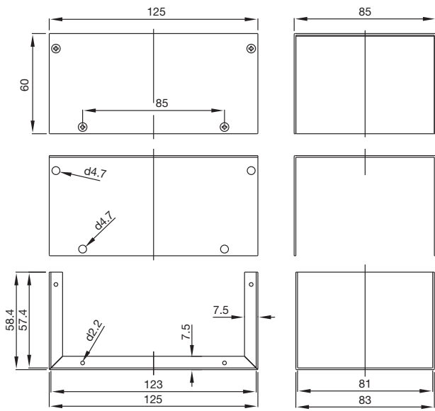
Minibox 31040108
