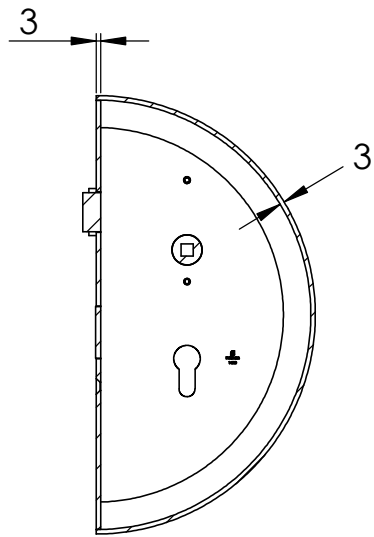
SCHNITT A-A
