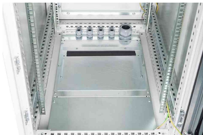
19" Industrie-Netzwerkschrank, Detailsicht
