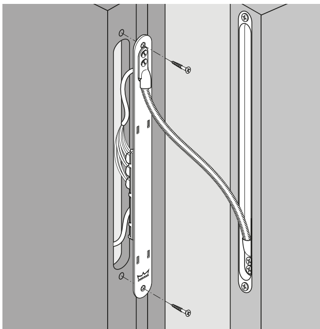
Lösbare Kabelübergangsstückverbindung LK 12
