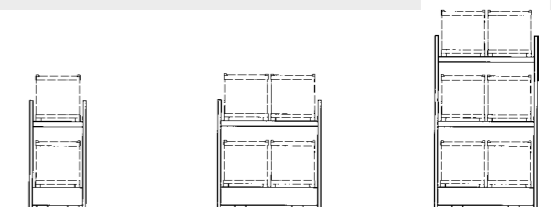
Combi-Regal Typ 3 K2-I, Grundfeld mit lackierter Auffangwanne, Bestell-Nr. 201-876-J9
