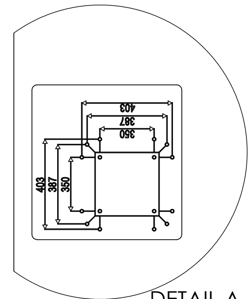
DETAIL A MAßSTAB 1 : 2
