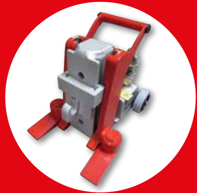
Hebegerät mit Sonderaufnahme/Sonderlasche
