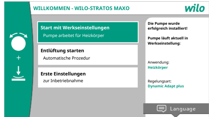
Fig. 1: Ersteinstellungsmenü
