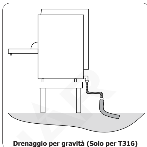
Drenaggio per gravità (Solo per T316)
