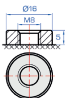
F12 (Schraubanschluss M8)
