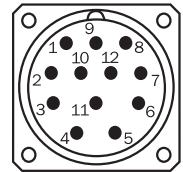
Ansicht Gerätestecker M23 am Encoder
