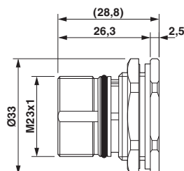
Maßzeichnung
