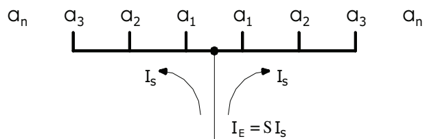
Einspeisung im Verlauf der Schiene oder Mitteleinspeisung
