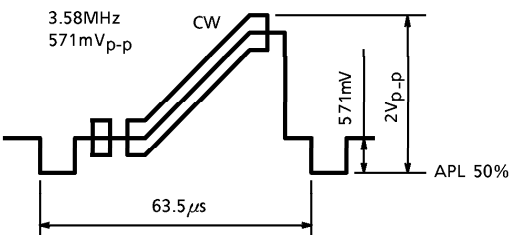
入力波形
