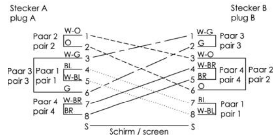
Schaltbild / Connection Diagram
