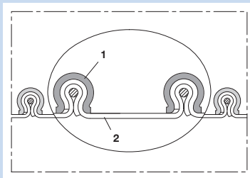
Wąż PVC z profilem zaciskowym, (do +120°C)
