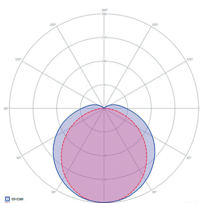
rozsył światła: opcja D02
