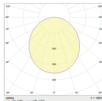
rozsył światła: opcja D03
