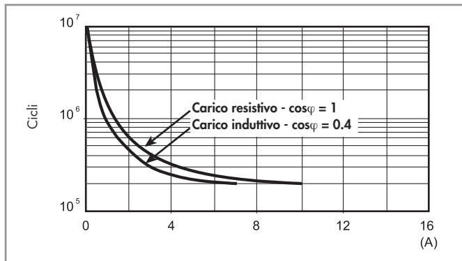
F 60 - Durata elettrica (AC) in funzione della corrente
