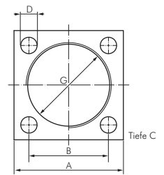
axiale Befestigung
