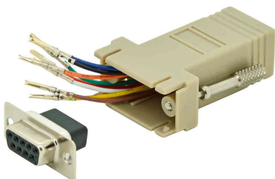
Adaptateur femelle RS 232 - femelle RJ45
