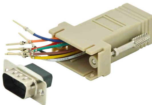
Adaptateur mâle RS 232 - mâle RJ45
