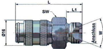
Außengewinde
