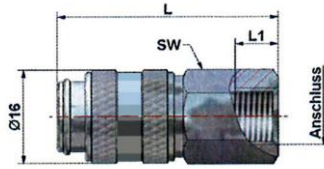
Innengewinde
