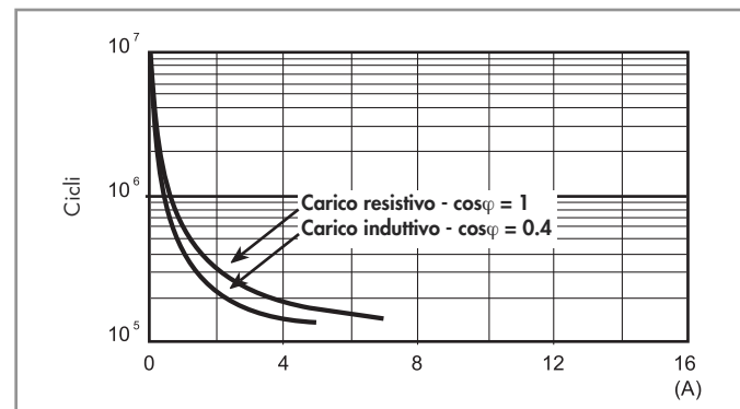
F 55 - Durata elettrica (AC) in funzione della corrente 4 contatti
