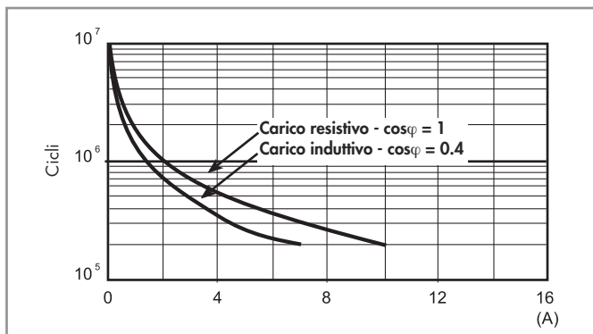
F 55 - Durata elettrica (AC) in funzione della corrente 2 e 3 contatti
