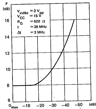
NOISE FACTOR F = f(a) FACTEUR DE BRUIT F = f(a)
