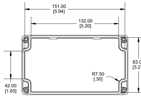
INSIDE LID
