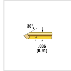
POGO-25A-S
