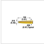
POGO-25Z
