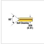
POGO-25Z1
