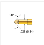
POGO-25L36-S
