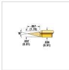
POGO-25Z-S
