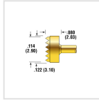
POGO-25T
