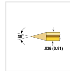
POGO-25L-S
