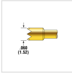
POGO-25L18
