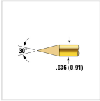
POGO-25L
