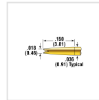
POGO-25V-S
