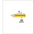
POGO-25B-S
