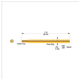
SPR-25W-1
