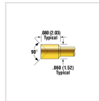
POGO-25J-S
