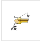
POGO-25A
