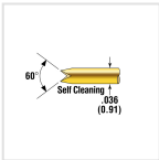
POGO-25UN-S
