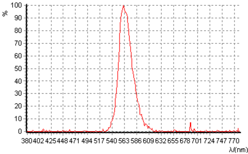
波长 Wavelength
