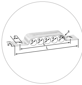
NORMAFIX® BSL TYP 512 FÜR 5 LEITUNGEN (GEMÄSS DIN 72573)
