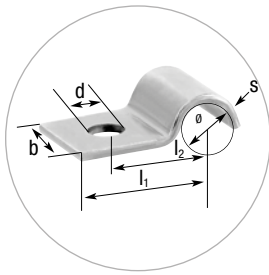
NORMAFIX® BSN TYP 520 FÜR 1 LEITUNG
