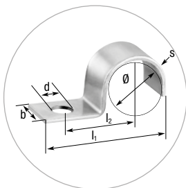
NORMAFIX® BSL TYP 510 FÜR 1 LEITUNG (gemäß DIN 72571)
