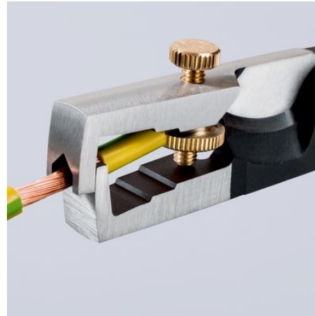
Geen onvrijwillige verstelling door borging met borgmoer
