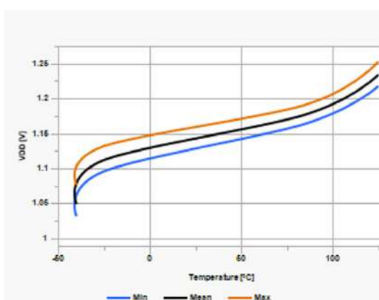
Figure 42-51. POR Rearm Voltage
