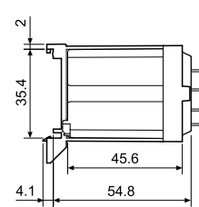
062.07 con relè
