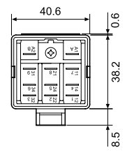
062.07 con relè
