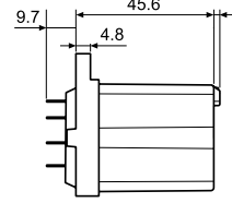
062.10 con relè
